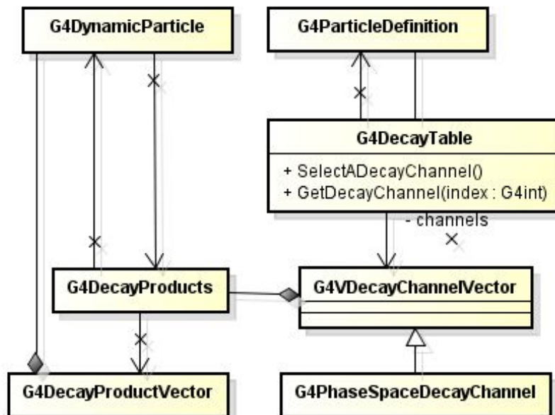
Fig. 2.20: Decay Table
