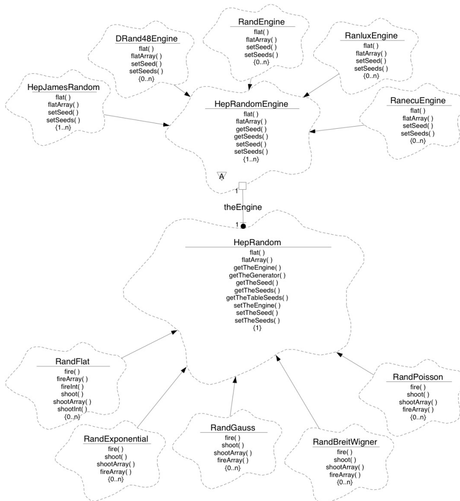
Fig. 2.24: HEPRandom module
